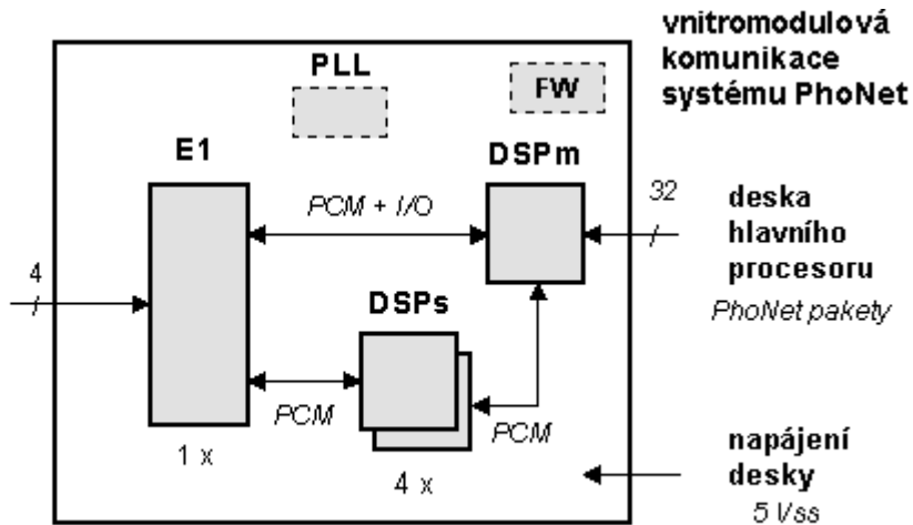
deska digitálního svazku PCM 2 Mbps
